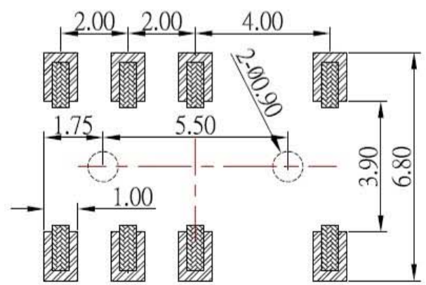
P.C.B LAND PATTERN
