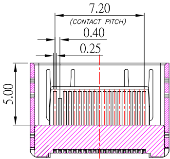
SECTION A-A SCALE 4:1
