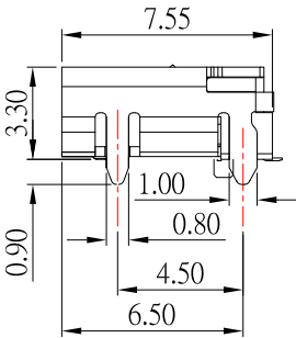
SECTION A-A SCALE 4:1
