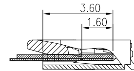
CABLE INSERT DIM.
