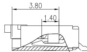
CABLE INSERT DIM. SECTION: A-A
