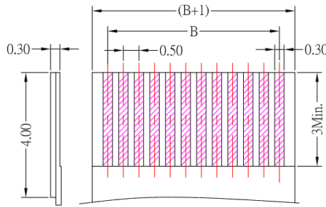
APPLI CABLE FPC
