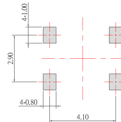
P.C.B LAND DIMENTION
