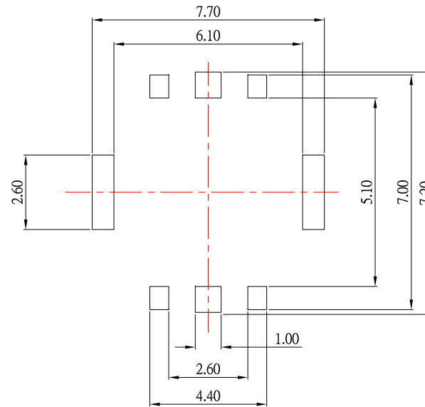
P.C.B LAYOUT
